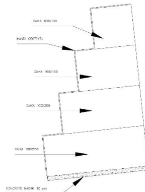
DETALHE 5 esc: 1/20
