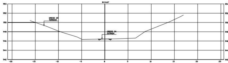
PERFIL TRANSVERSAL SESSÃO 8+14,67 esc: 1/100
