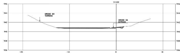
PERFIL TRANSVERSAL SESSÃO 3+0.00 esc: 1/100
