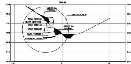
PERFIL TRANSVERSAL SESSÃO 12+6,69 esc: 1/100
