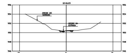
PERFIL TRANSVERSAL SESSÃO 12+16,23 esc: 1/100
