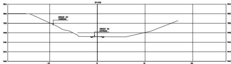
PERFIL TRANSVERSAL SESSÃO 10+0,00 esc: 1/100
