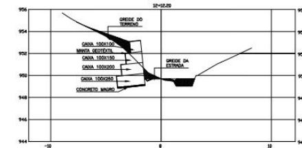
PERFIL TRANSVERSAL SESSÃO 12+12,20 esc: 1/100
