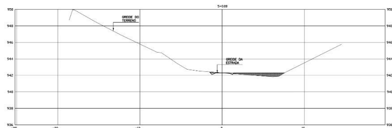
PERFIL TRANSVERSAL SESSÃO 5+0.00 esc: 1/100
