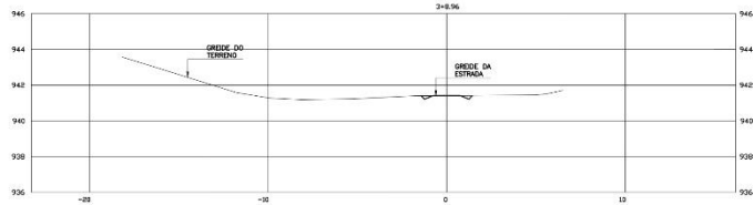
PERFIL TRANSVERSAL SESSÃO 3+8.96 esc: 1/100
