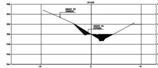
PERFIL TRANSVERSAL SESSÃO 12+0,00 esc: 1/100
