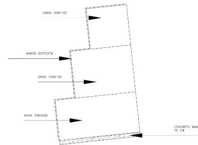
DETALHE 2 esc: 1/20
