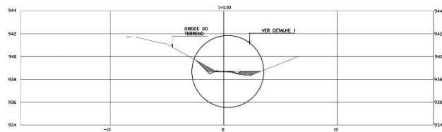
PERFIL TRANSVERSAL SEÇÃO 1+0,00 esc: 1/100
