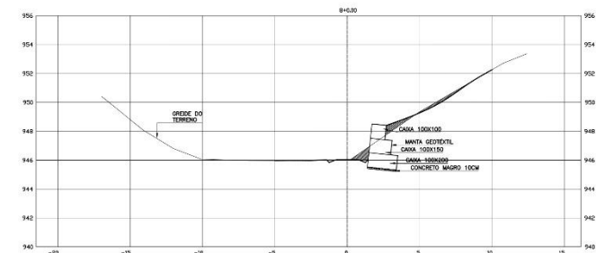
PERFIL TRANSVERSAL SESSÃO 8+0.00 esc: 1/100
