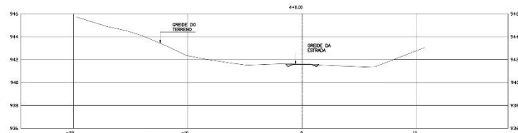
PERFIL TRANSVERSAL SESSÃO 4+0.00 esc: 1/100
