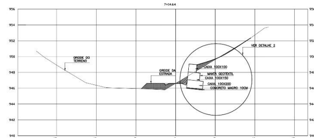
PERFIL TRANSVERSAL SESSÃO 7+14.64 esc: 1/100
