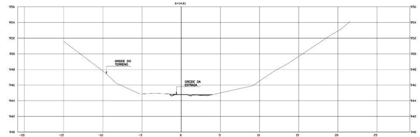
PERFIL TRANSVERSAL SESSÃO 6+14.61 esc: 1/100
