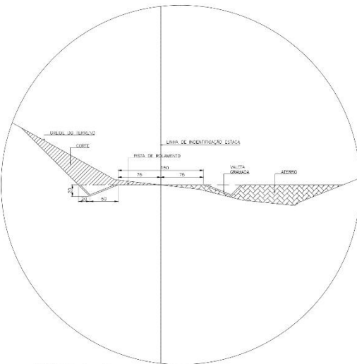
DETALHE 1 esc: 1/20
