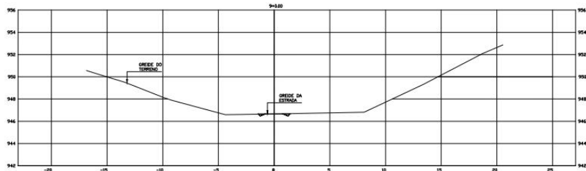
PERFIL TRANSVERSAL SESSÃO 9+0,00 esc: 1/100
