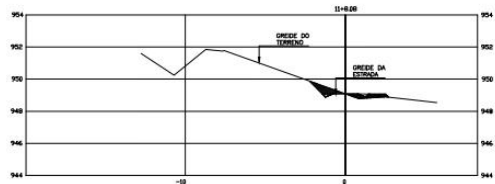
PERFIL TRANSVERSAL SESSÃO 11+8,08 esc: 1/100
