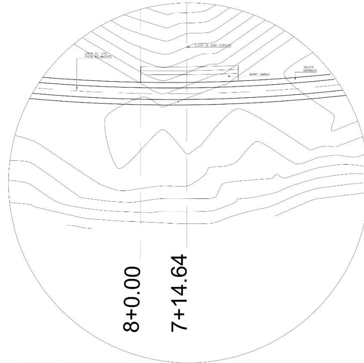
DETALHE 4 - PLANTA MURO GABIÃO esc: 1/100
