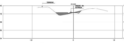
PERFIL TRANSVERSAL SEÇÃO 2+0,00 esc: 1/100
